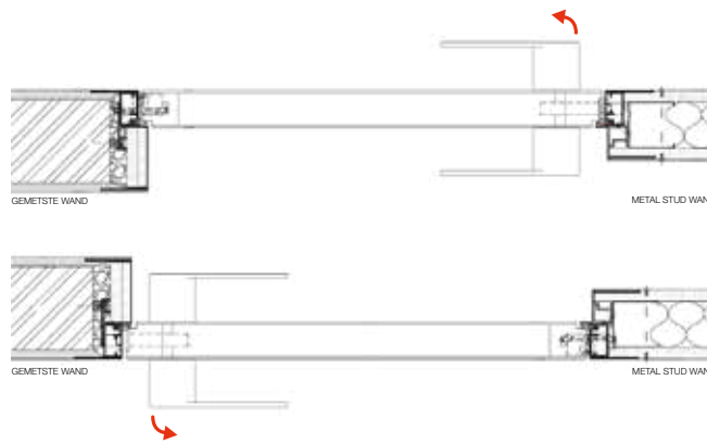
INSTALLATIE TREKKEND EU RECHTS
