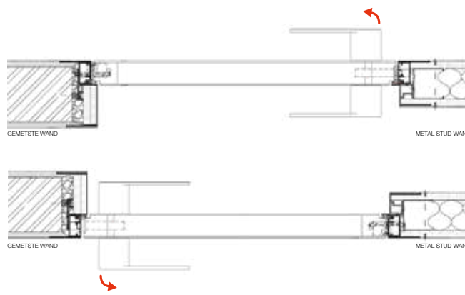
INSTALLATIE TREKKEND EU RECHTS
